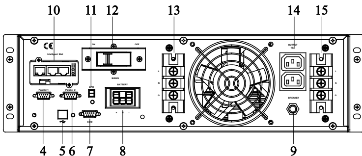
Tampak Belakang
