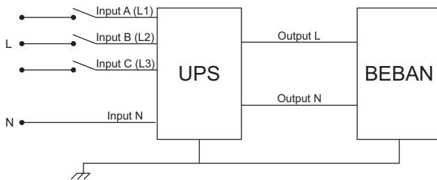
Tiga fase input, satu fase output
