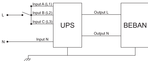
Satu fase input, satu fase output
