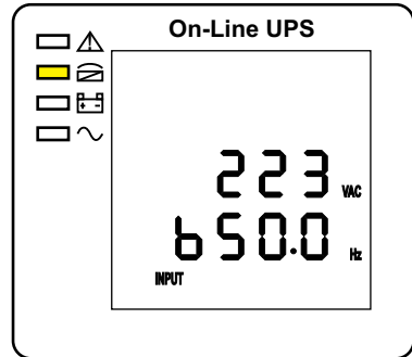
3. Input/ Frekuensi fase B (L2)
